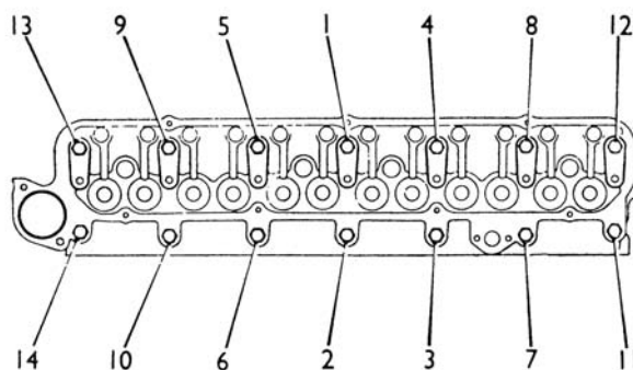
Anziehfolge Zylinderkopfschrauben / Sequence for head bolts
