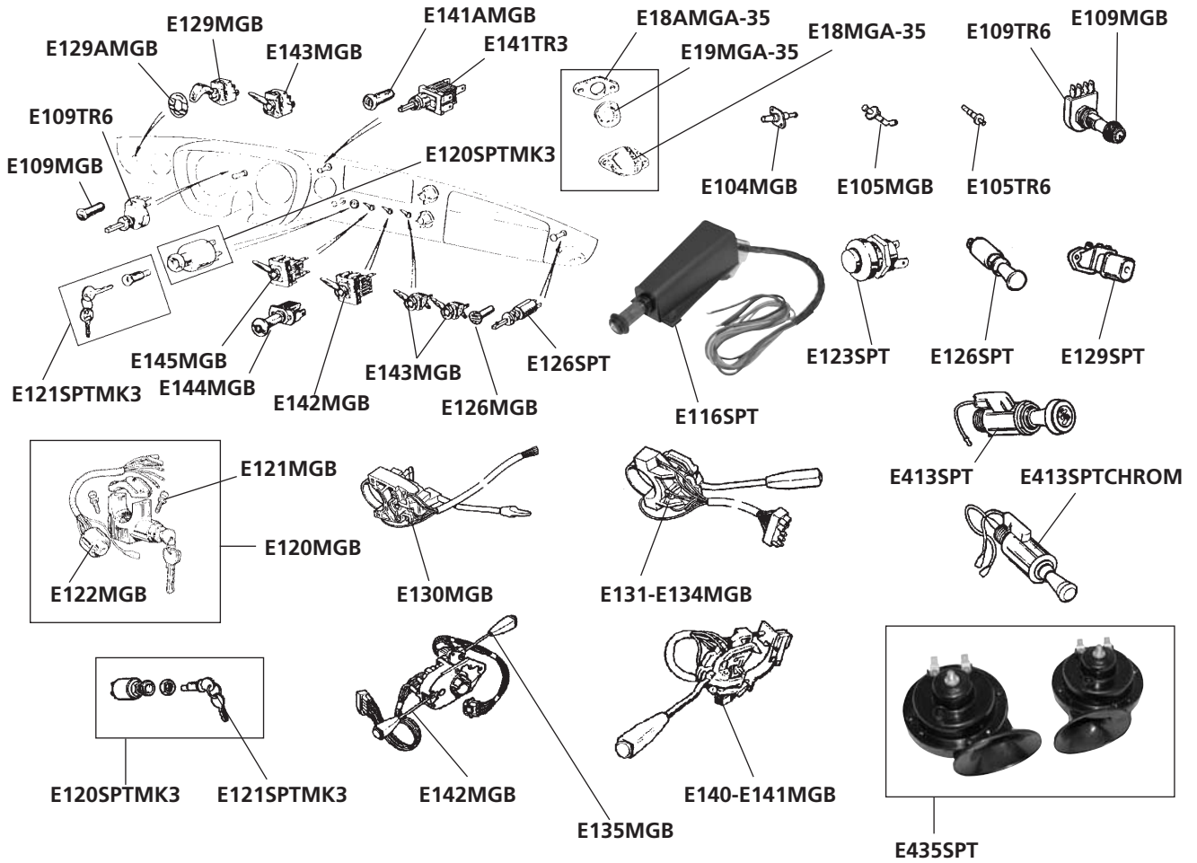
Schalter Armaturen Brett / Switches instrument panel 1972-76 bis / up to GHN/D5 41000
