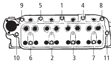
Anziehfolge Zylinderkopfschrauben / Sequence for head bolts
