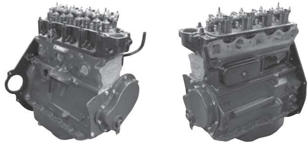
Abb. 4-Zyl. / Fig. 4-cyl.
